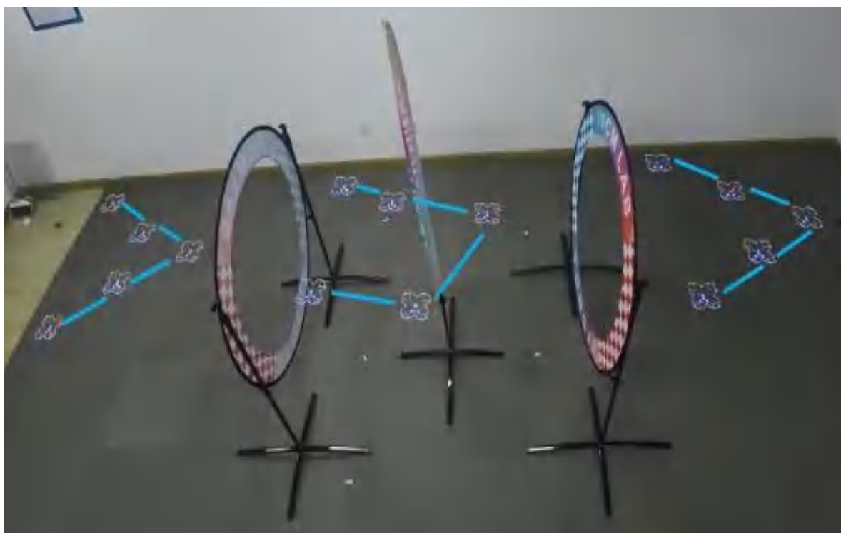
图 2.1 多智能体编队导航实验
