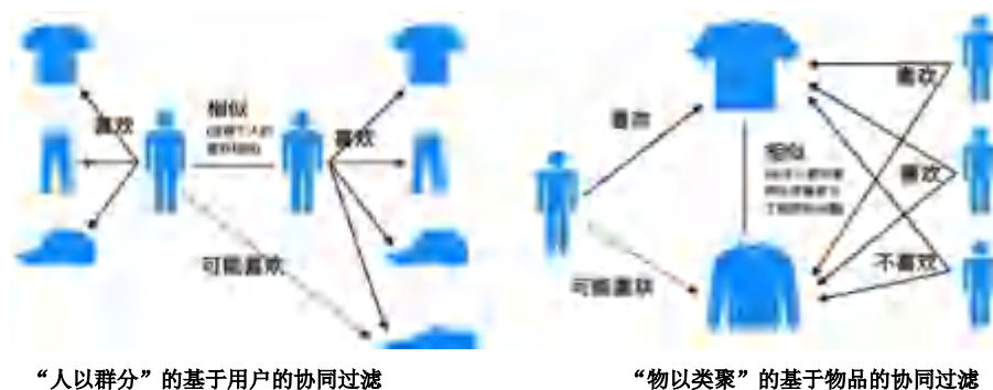
图 3.3 两种协同过滤算法对比
