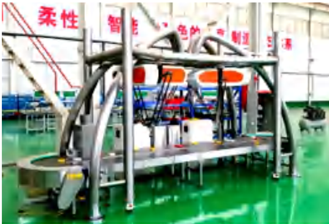
图 2.2 高速多并联机器人协同作业系统应用场景图
