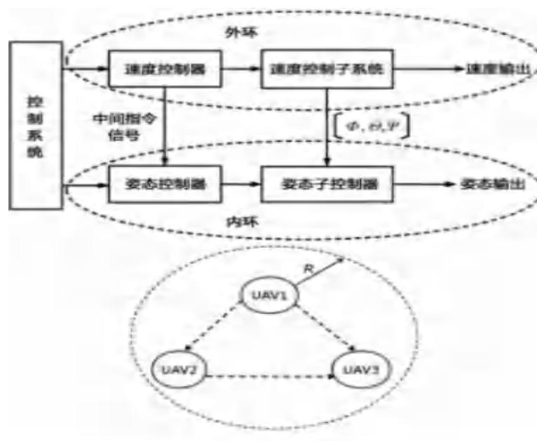
图 3.2 分布式算法
