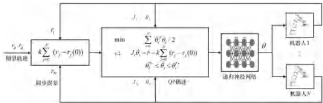
图 5.15 多机器人智能协同控制框图
