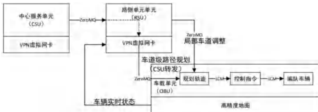
图 5.5 网联式自动驾驶车辆控制流程
