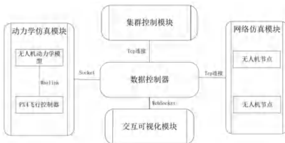
图 5.13 数据控制器智能协同控制框图
