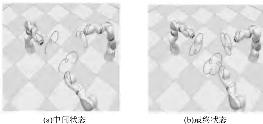
图 5.16 V-REP 环境下对三环曲线的跟踪效果
