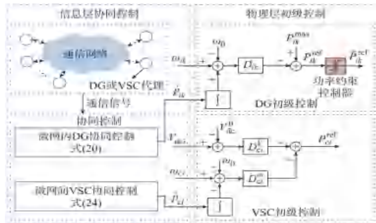
图 2.4 柔性直流互联孤岛微网群分布式频率控制器
