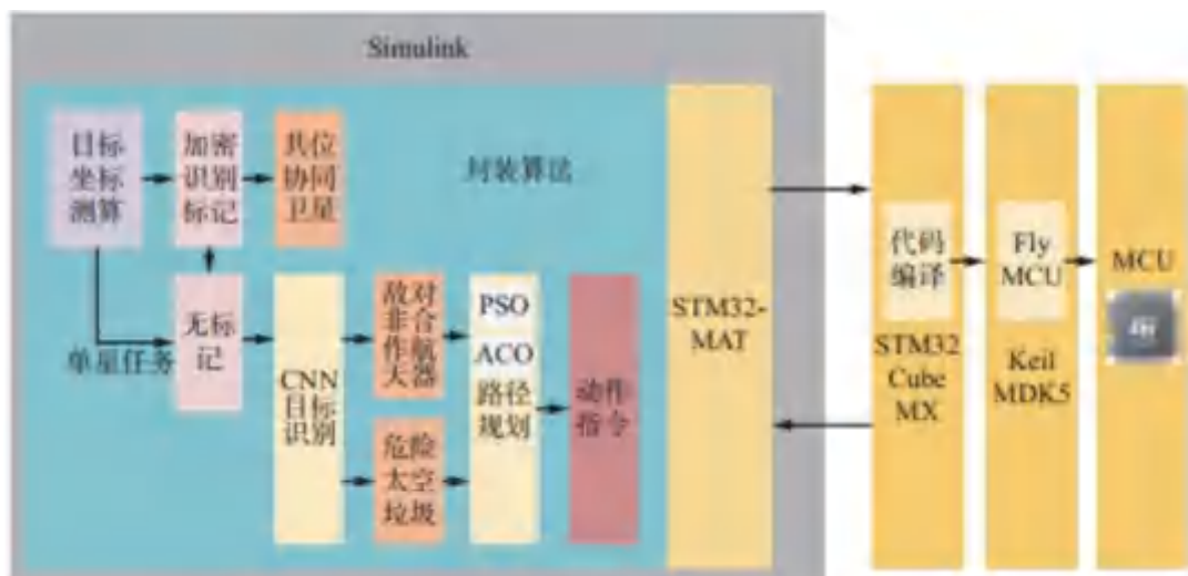
图 5.14 智能协同控制关键技术地面验证平台架构
