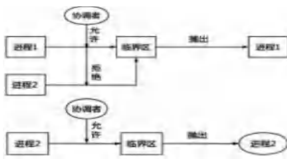
图 3.1 集中式算法
