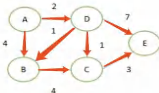
图 3.8 最短路径
